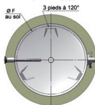
DÉTAIL PLATEAU
